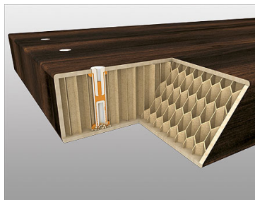
Зафиксированный дюбель
